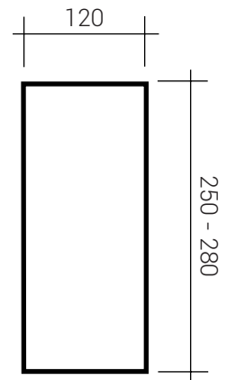
Bordstein ohne Anlauf „B6“ ca. Gewicht 85 kg /lfm
