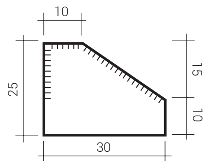
Flachbord „F15“ ca. Gewicht 200 kg/lfm
