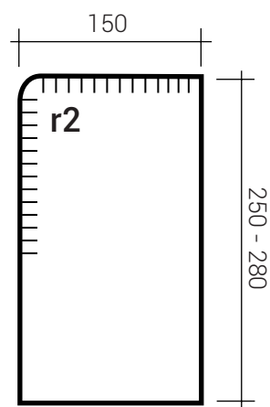
Rundbord „B6“ ca. Gewicht 135 kg /lfm
